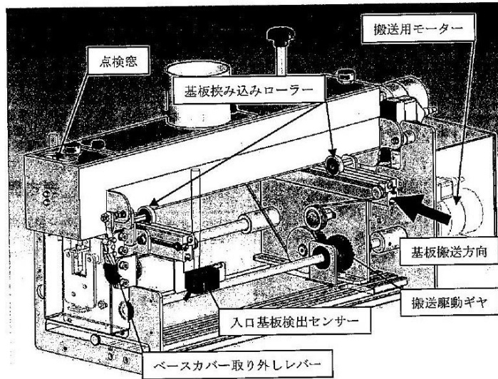
写真1-1：クリーニングユニット各部名称
